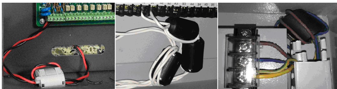
图2 不符合认证产品一致性的临时性磁环连接方式
