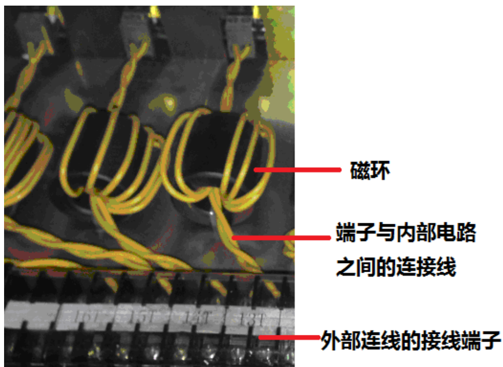
图 1 在端子与内部电路之间安装磁环示例
